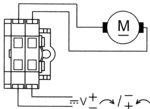
D.c.
