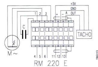
Monofase con tachimetrica 1-phase with tacho
