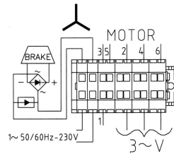
Trifase con freno a stella Star 3-phase with brake
