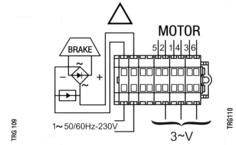
Trifase con freno a triangolo Triangle 3-phase with brake
