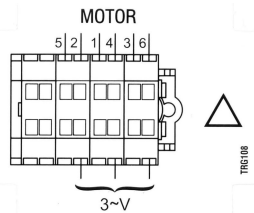
Trifase a triangolo Triangle 3-phase
