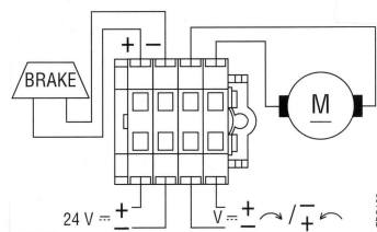
D.c. con freno D.c. with brake
